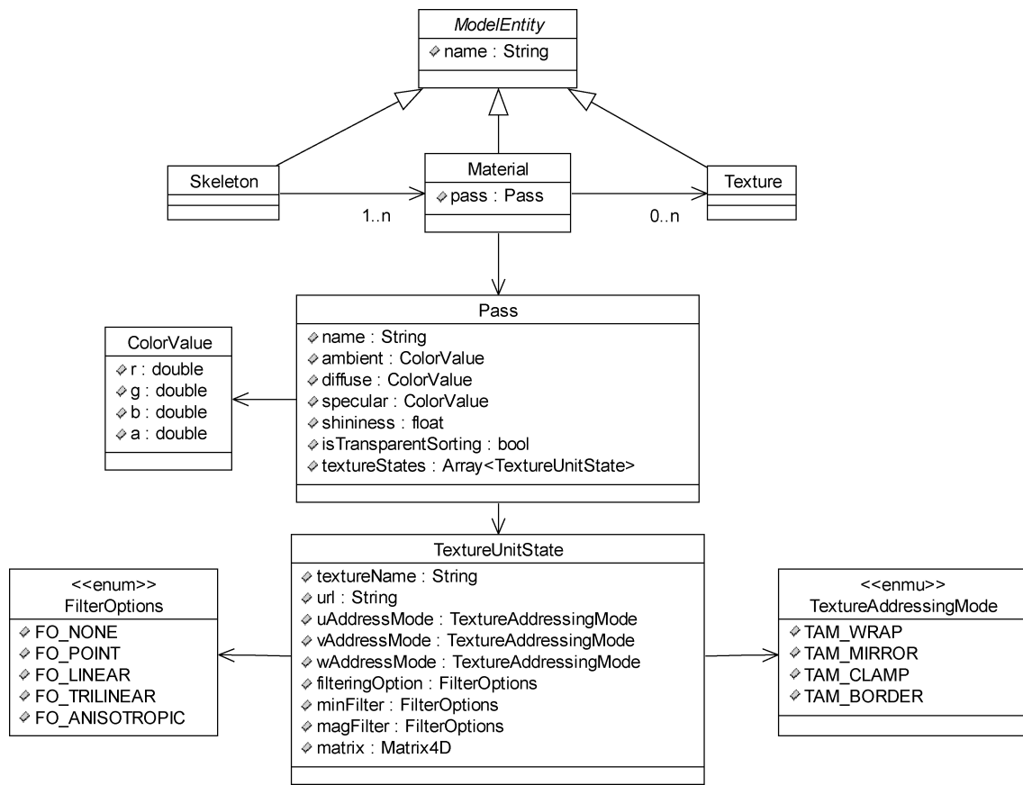
图 5 材质对象 UML 图
