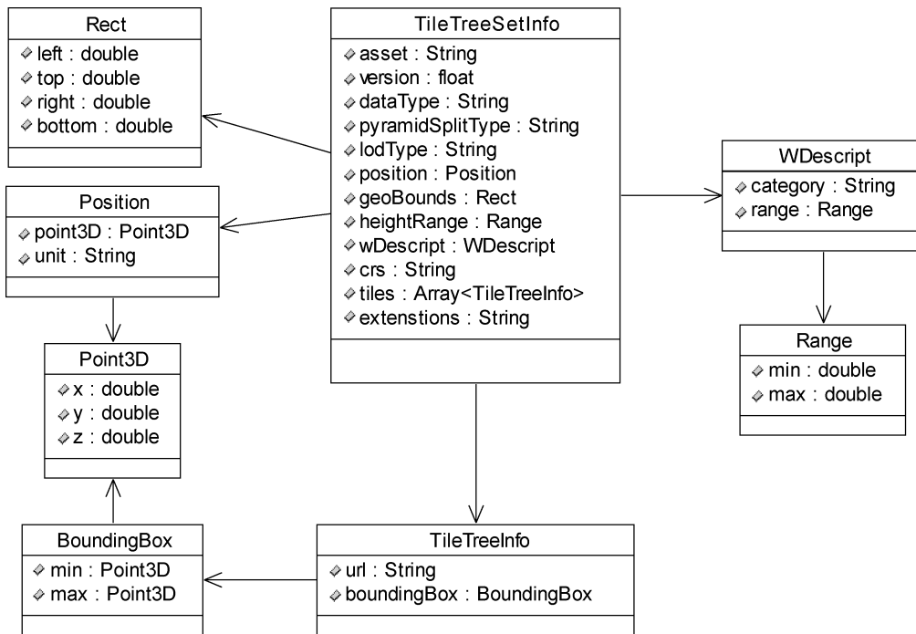
图 2 描述文件的 UML 图
