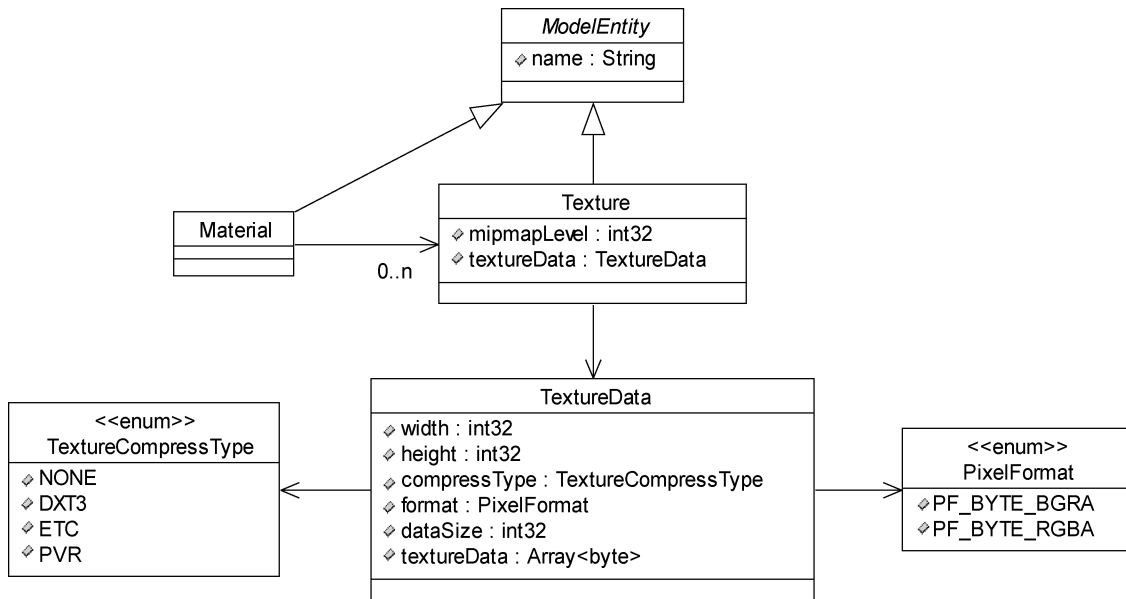
图 6 纹理对象 UML 图
