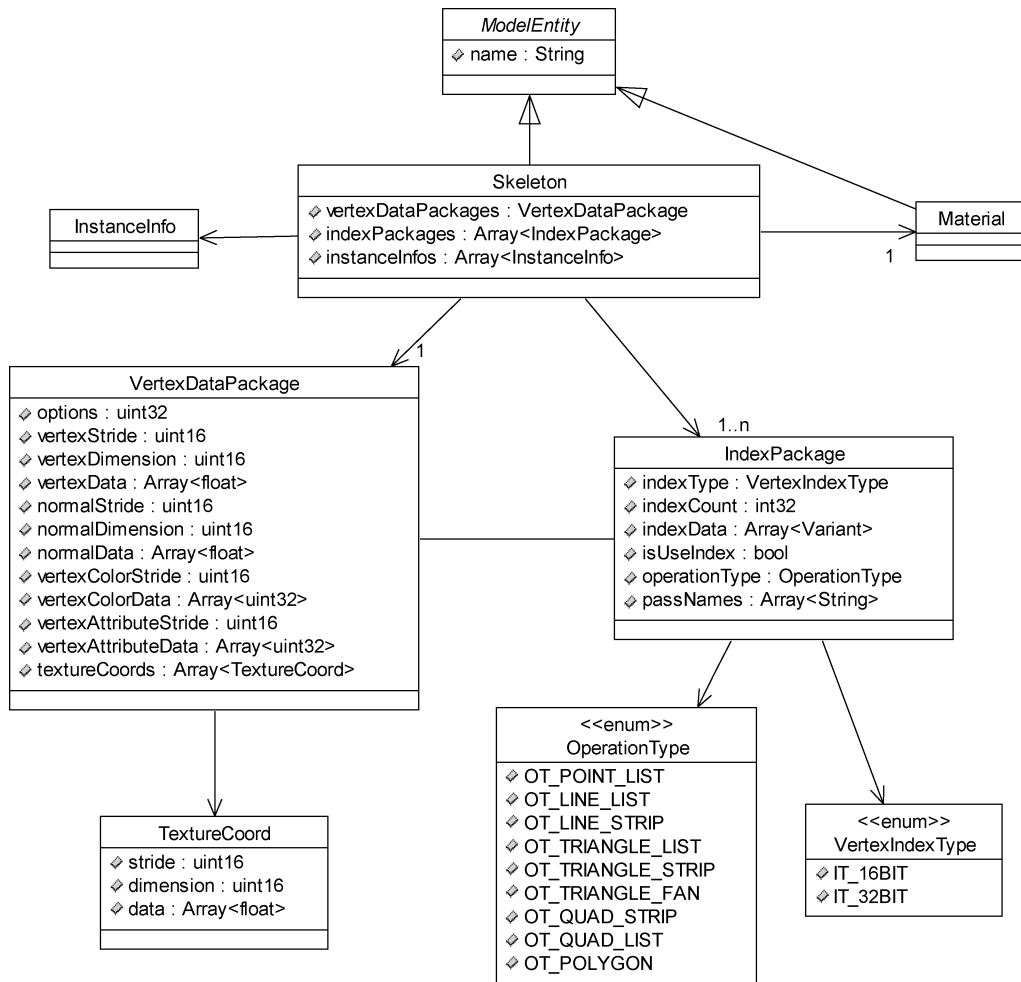
图 4 骨架对象 UML 图
