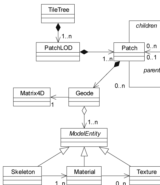
图 1 树形结构 UML 图
